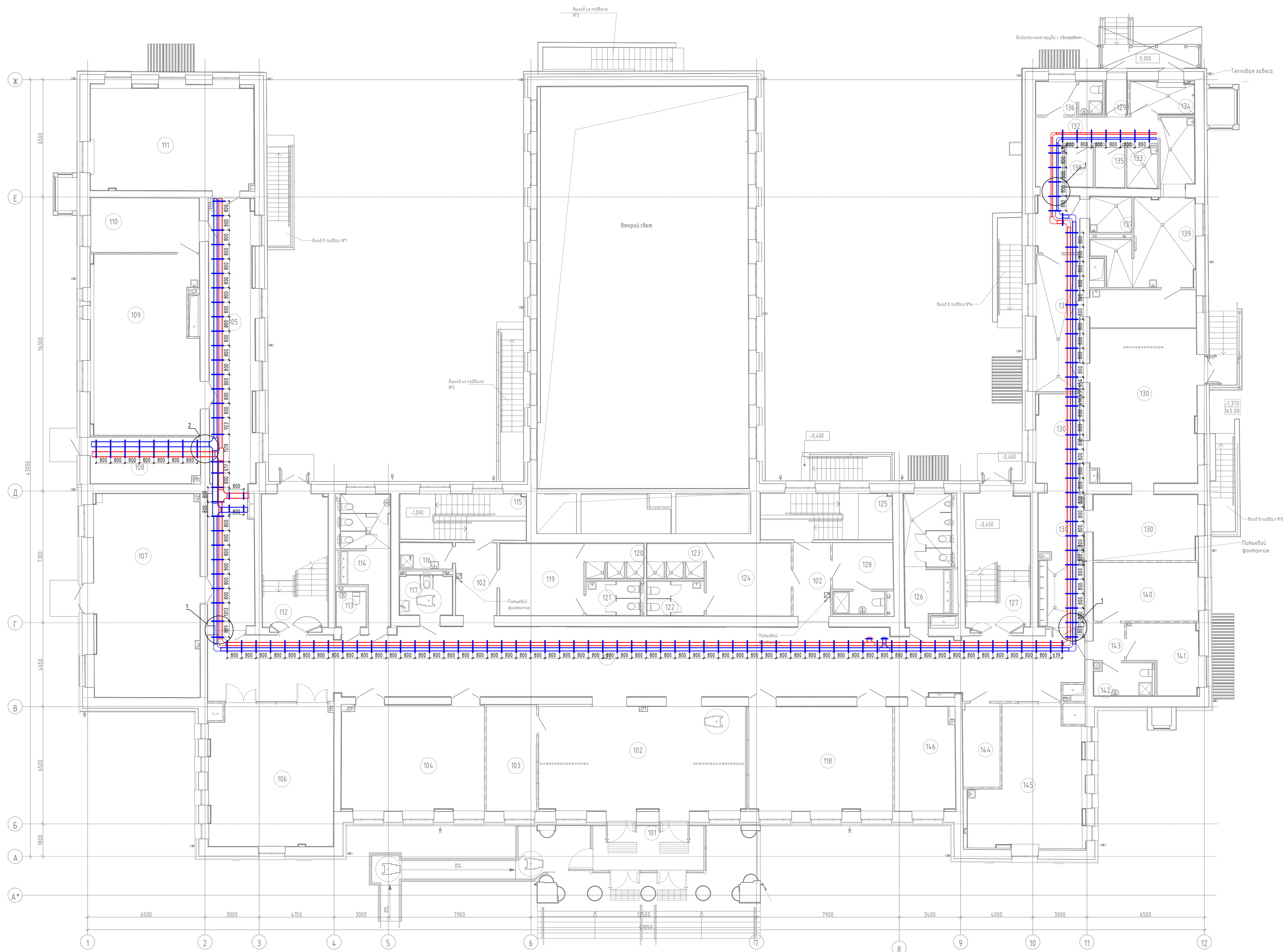
План 1 этажа
